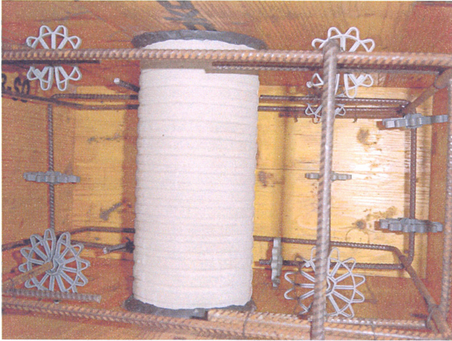
Bild 1: Horizontal ausgerichtete PSI FZ-Mauerhülse DN 100 vor dem Betonieren des Prüfkörpers
