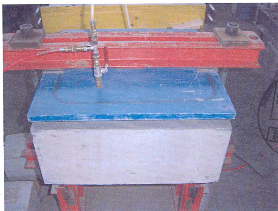
Bild 2: Prüfkörper während der Dichtigkeitsprüfung
